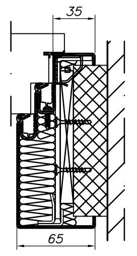
MASSIEVE WAND DUBBELE SPONNING
