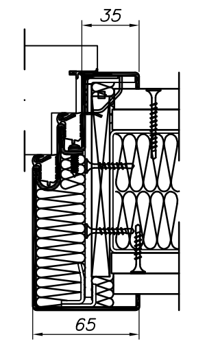
METAL-STUD WAND DUBBELE SPONNING
